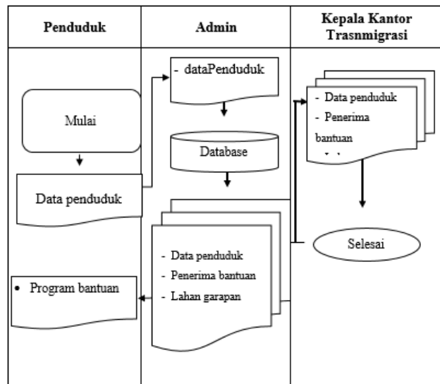
Gambar 3.4. Diagram Arus Data Sistem Yang Diusulkan
